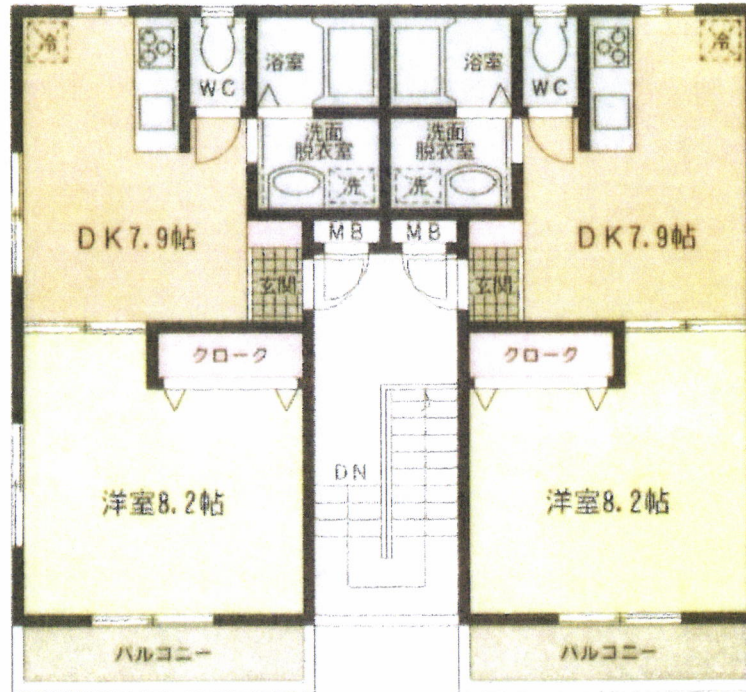
2階平面図
